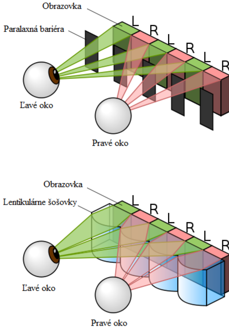
Obr. 7.45 Princíp paralaxovej bariéry
